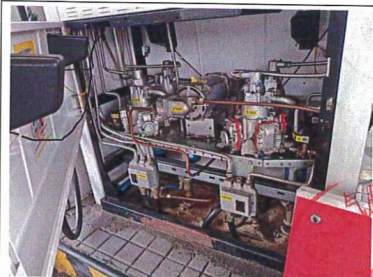
加油机内部
