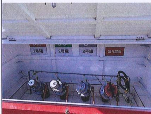
卸油口
