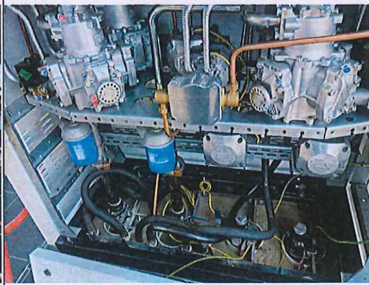
加油机内部
