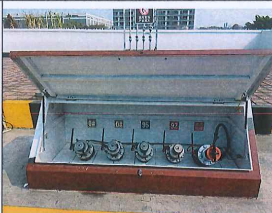
卸油口
