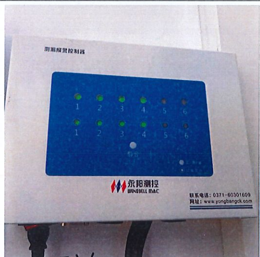
双层油罐--双层油管渗漏监测系统
