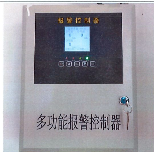
站房内可燃气体报警控制器
