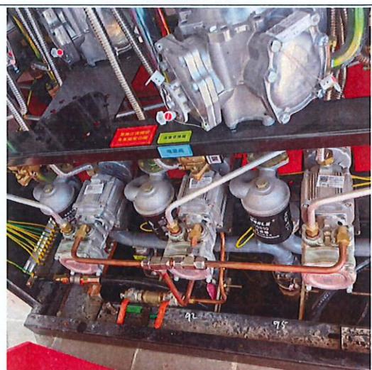
加油机内部
