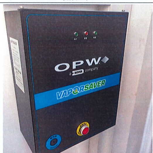
站房内三次油气回收装置控制器
