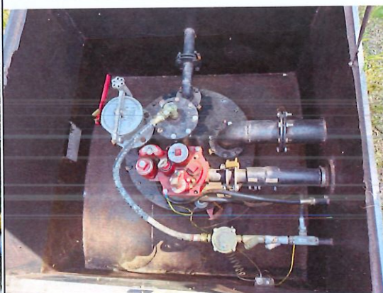
储罐操作井
