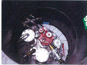
油罐操作井
