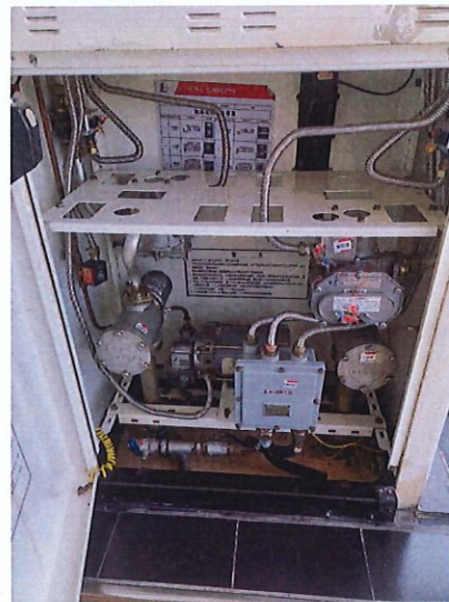
加油机内部
