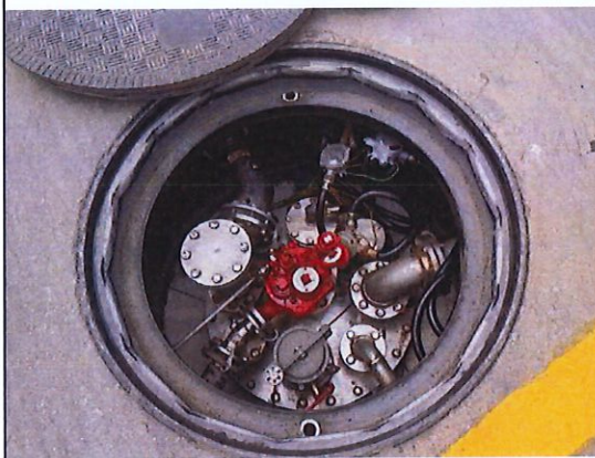
储罐操作井
