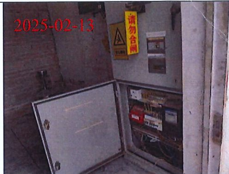
配电柜
