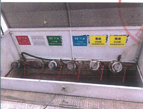
卸油口
