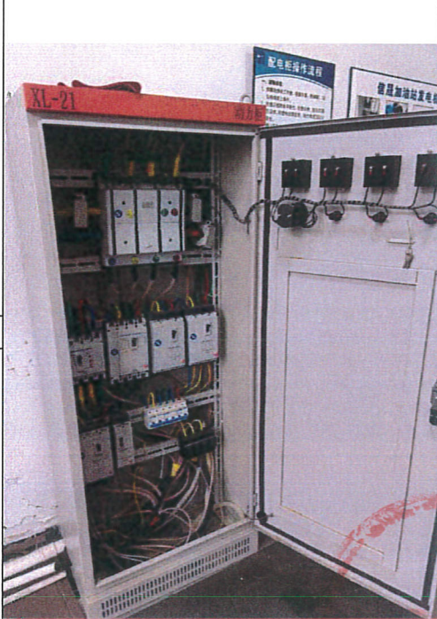
配电柜
