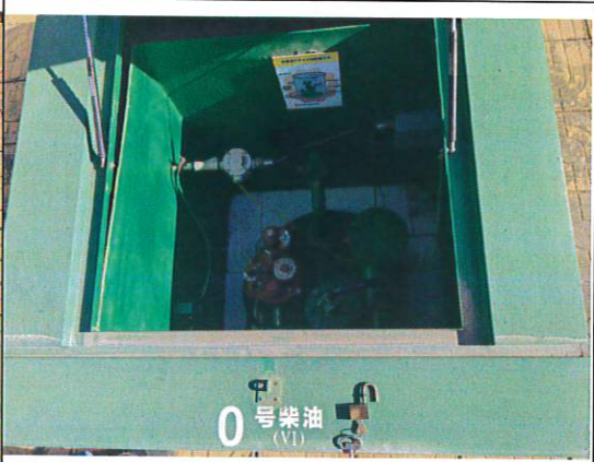
柴油储罐操作井
