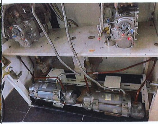
加油机内部
