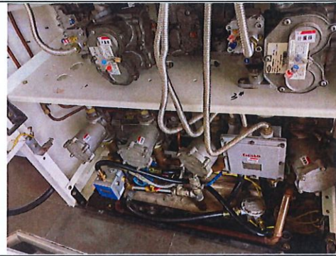
加油机内部
