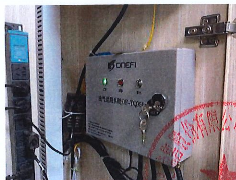
双层管道在线泄漏监测
