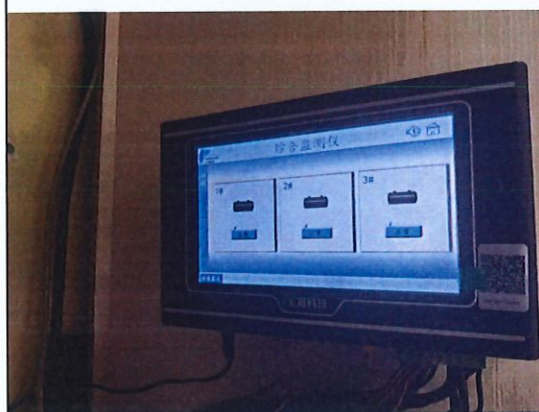
双层油罐在线泄漏监测系统
