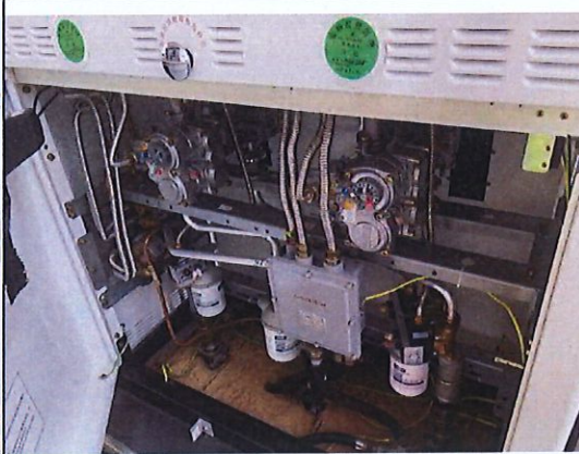
加油机内部
