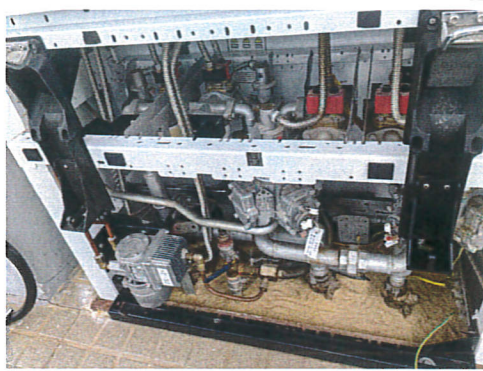
加油机内部
