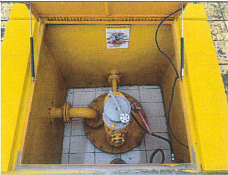
储罐操作井
