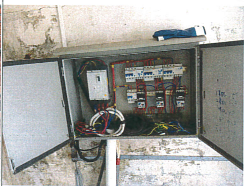
配电柜
