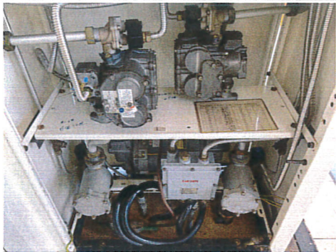
加油机内部
