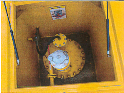
油罐操作井
