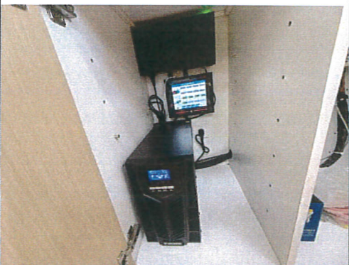
油管在线渗漏监测系统
