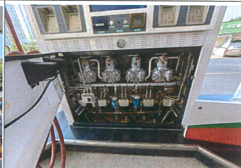
加油机内部
