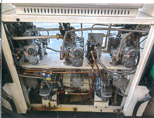
加油机内部
