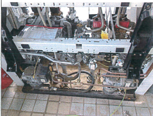
加油机内部
