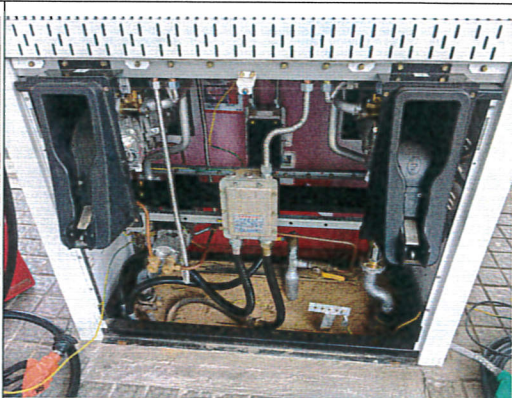
加油机内部
