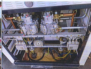
加油机内部
