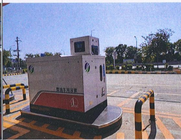
撬装尿素溶液加注装置
