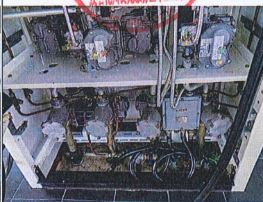
加油机内部
