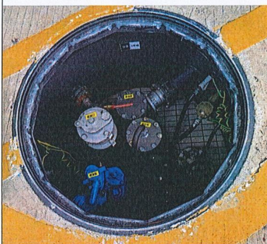
人孔操作井
