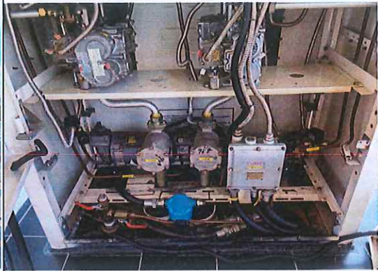
加油机内部
